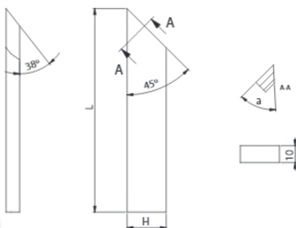
Rysunek przedstawia nóż lewy.
