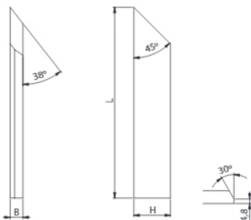
Rysunek przedstawia nóż lewy.
